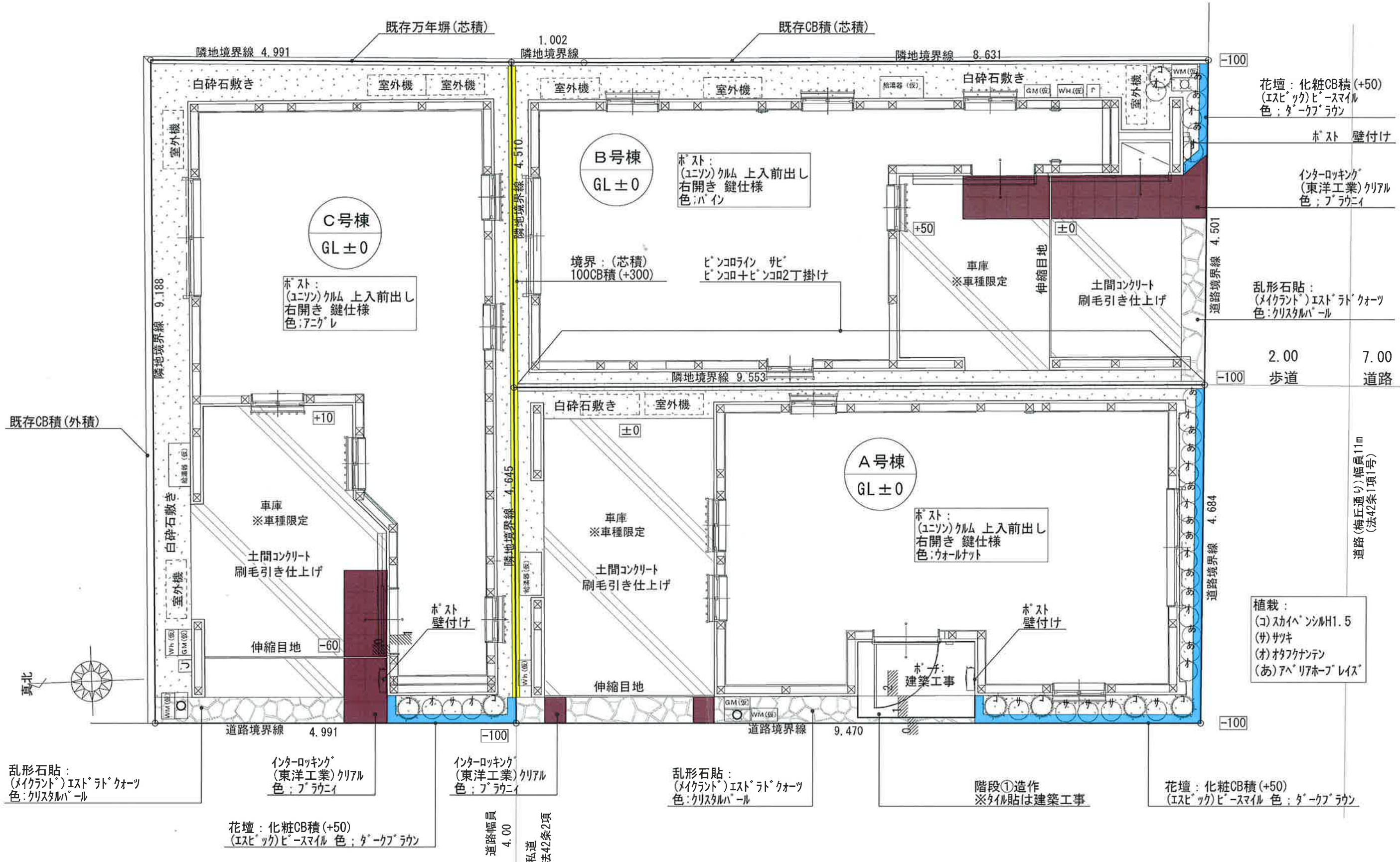
平面図 S : 1/50
